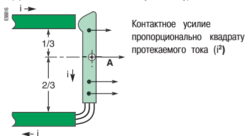
Усилия от протекаемого тока КЗ
