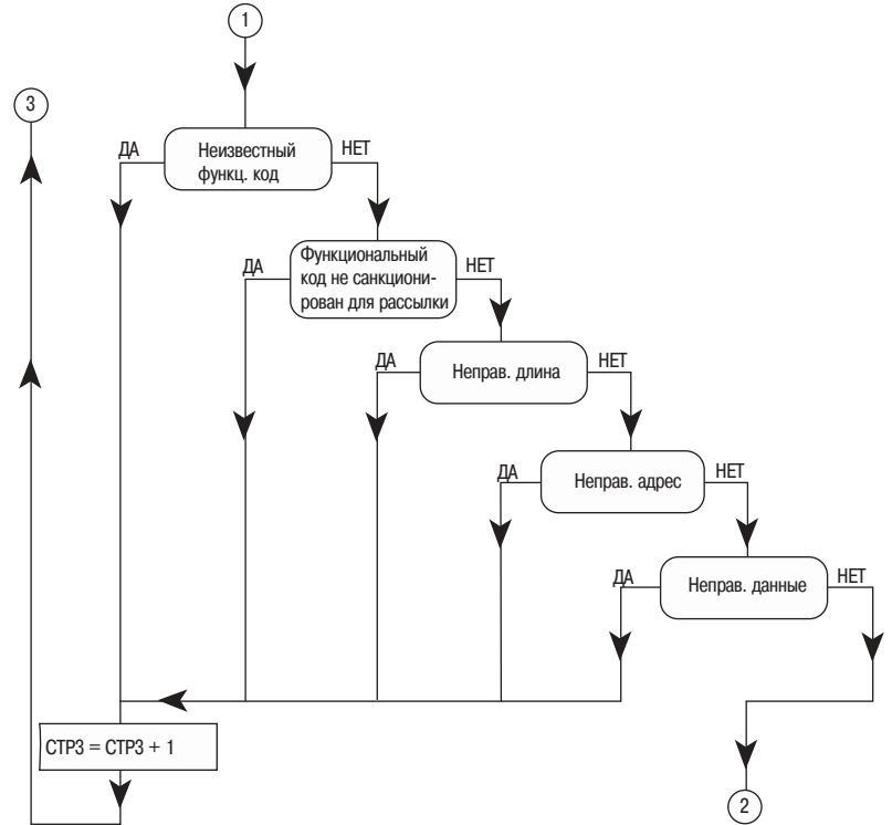
Алгоритм управления счетчиками (продолжение)
