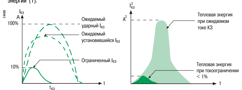
Токоограничение и снижение выделяемой тепловой энергии
