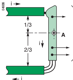
Усилия от протекаемых токов
