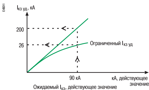
Кривая токоограничения
