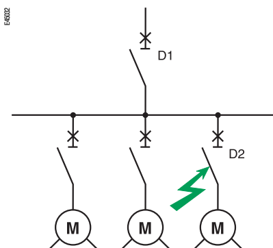
Селективность между выключателями для защиты электродвигателя
