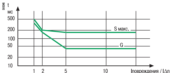
Время срабатывания G и S
