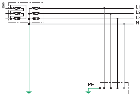
Система TT
