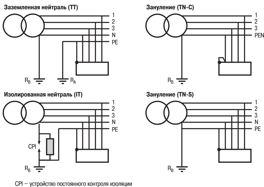
Рис. 6: Три принципиальные схемы заземления – ТТ, ТN, IT, установленные стандартом МЭК 60364-1. ТN может быть либо ТN-С (нейтраль и РЕ совмещены), либо ТN-S (нейтраль и РЕ разделены).
