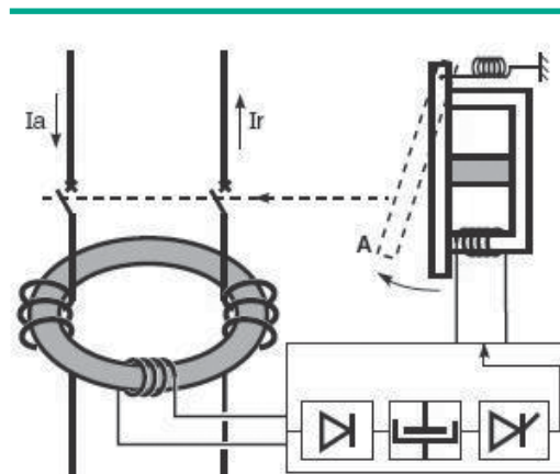
Рис. 11: через средство тора ток замыкания передает энергию сигнала электромагниту, якорь которого удерживается в притянутом состоянии с помощью постоянного магнита. Когда порог срабатывания достигнут, электромагнит нейтрализует силу притяжения постоянного магнита, якорь под действием пружины отходит от сердечника, приводит в движение контакты – выключатель отключается.
