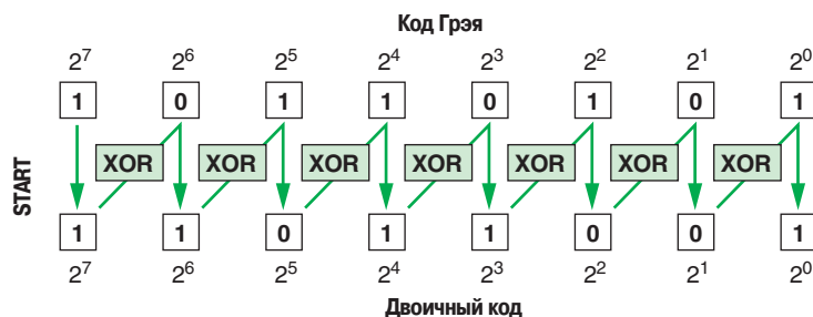
Рис. 54: Принцип конвертирования кода Грея в двоичный код
