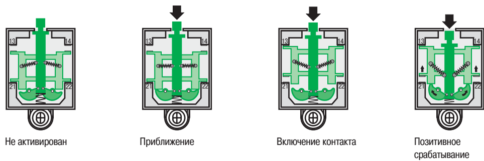
Рис. 3: Различные позиции контакта мгновенного действия
