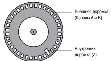
Рис. 47: Вид кодировочного диска инкрементального датчика углового положения
