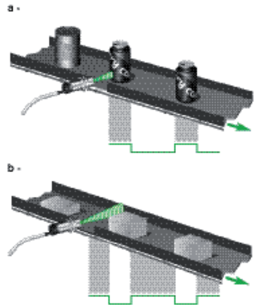
Рис. 27: Использование ультразвуковых датчиков: а/ бесконтактный или диффузный режимы; б/ рефлексный режим.
