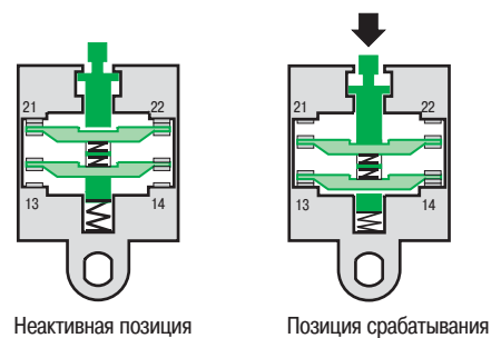
Рис. 4: Пример контакта медленного действия
