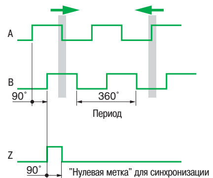
Рис. 48: Принцип определения направления вращения и сигнал синхронизации Z
