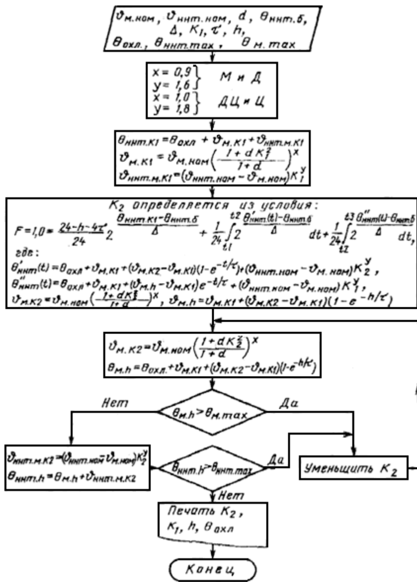
БЛОК-СХЕМА РАСЧЕТА ДОПУСТИМЫХ АВАРИЙНЫХ ПЕРЕГРУЗОК для трансформаторов классов напряжения до 110 кВ включительно*
