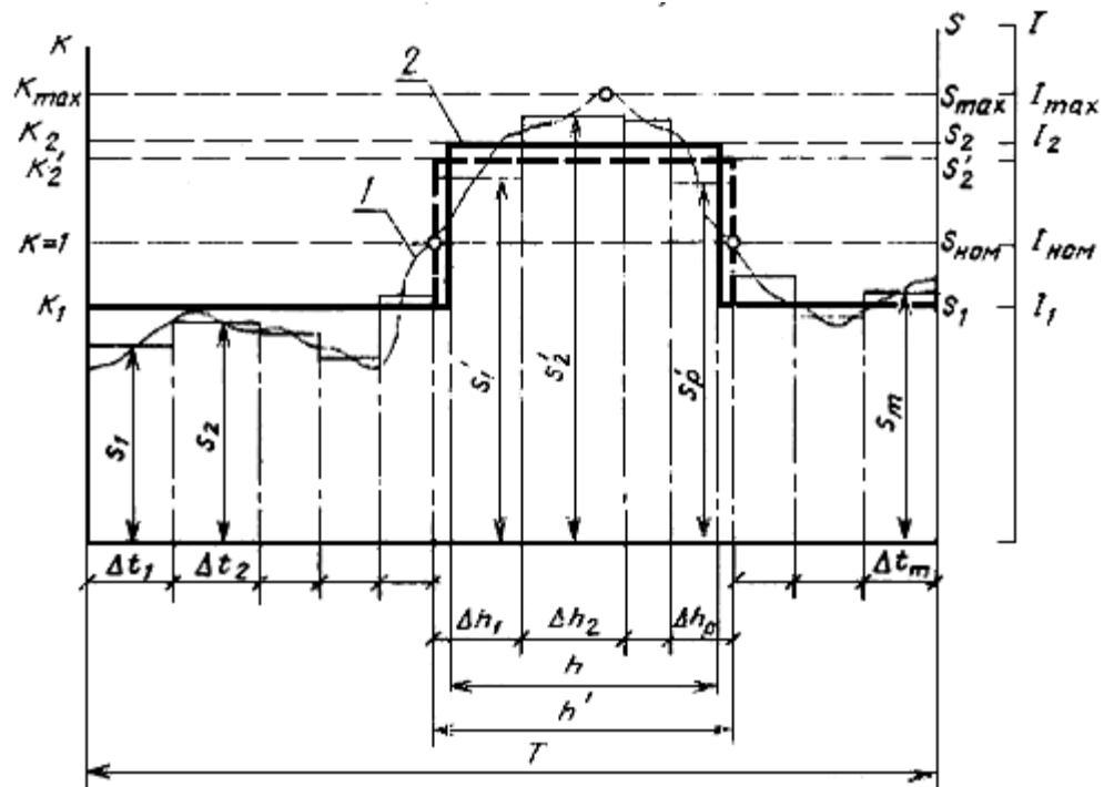
1 - исходный график нагрузки; 2 - двухступенчатый прямоугольный график нагрузки
