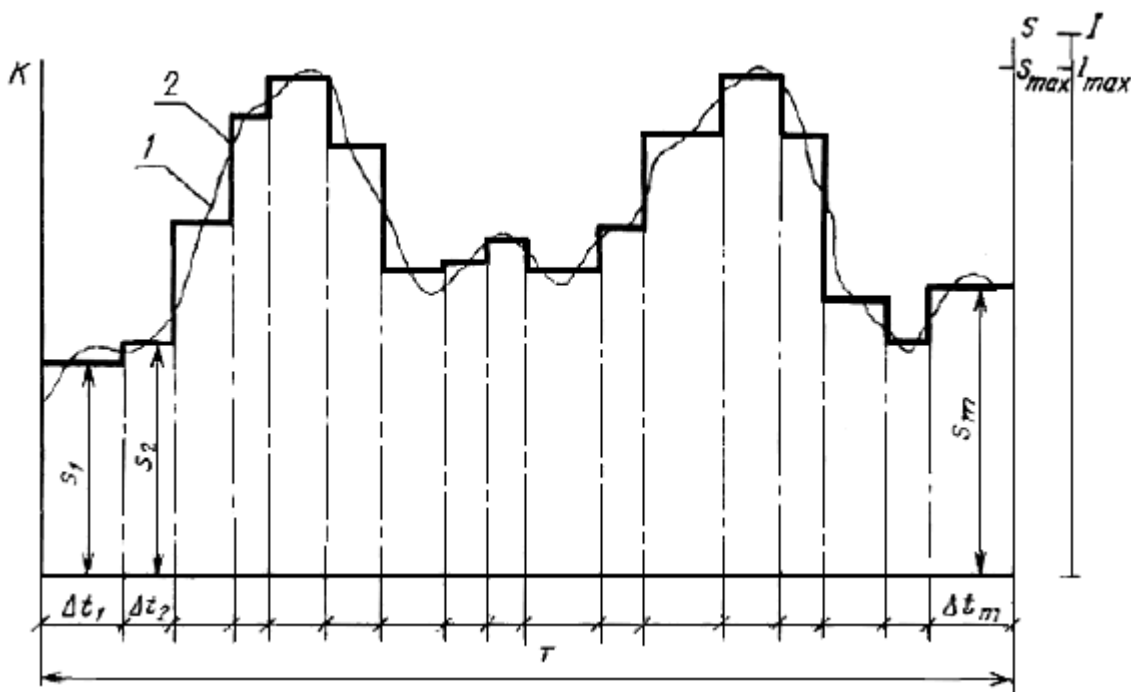
1 - исходный график нагрузки; 2 - эквивалентный прямоугольный график нагрузки
