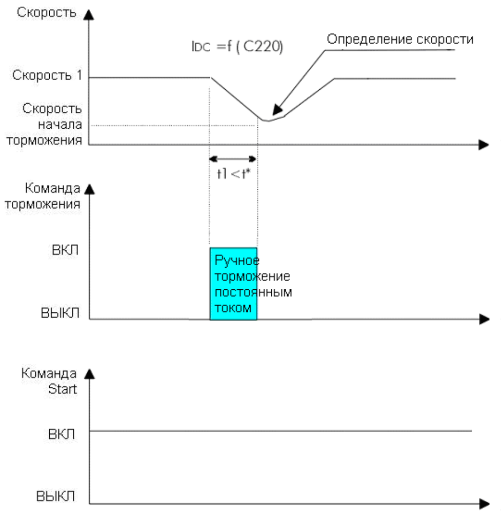
Рис. 56: Ручное торможение (Пример 3). Скорость, торможение, команда торможения и команда START при t1 < t^* и алгоритме управления IFD при включенной функции определения скорости.
