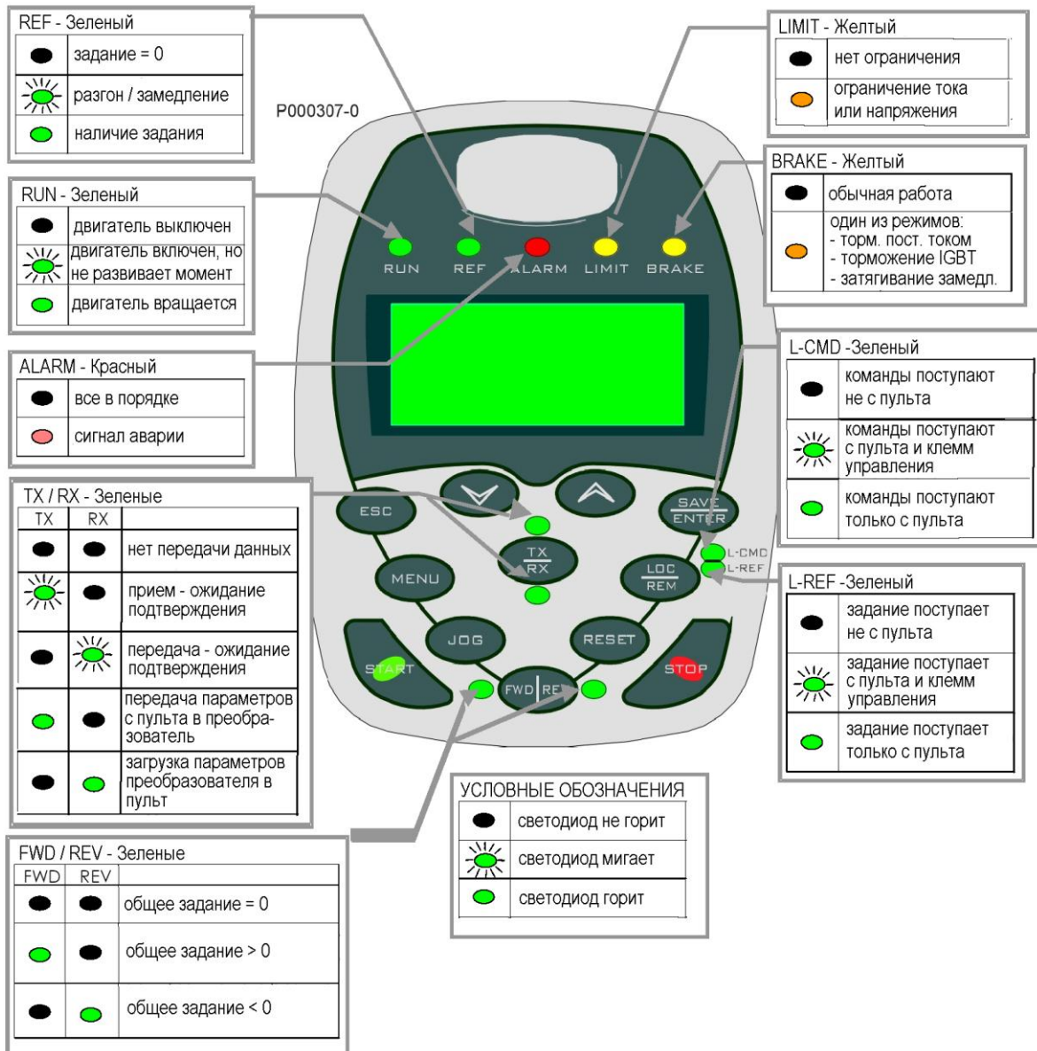
Рис. 3: Пульт управления
