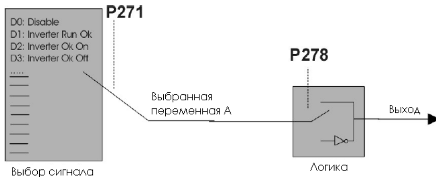
Рис. 32: Режим DIGITAL
