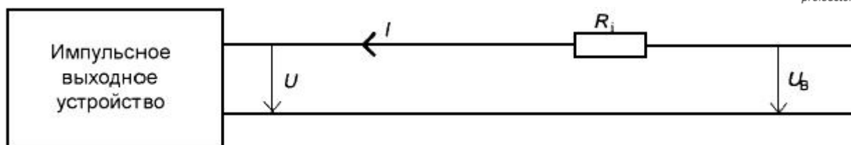
Рисунок Е.2 - Испытательная схема импульсного выходного устройства
