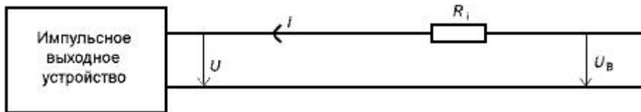
Рисунок С.1 - Испытательная схема импульсного выходного устройства
