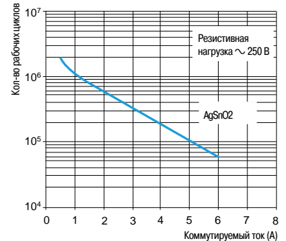
Электрическая износостойкость
