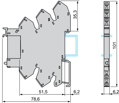
RSL 1PR●● с пружинными клеммами
