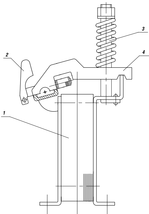
Рисунок 2. Расцепитель электромагнитный
