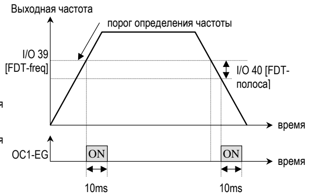
[Выход OC1 определен как 'FDT-PULSE']
