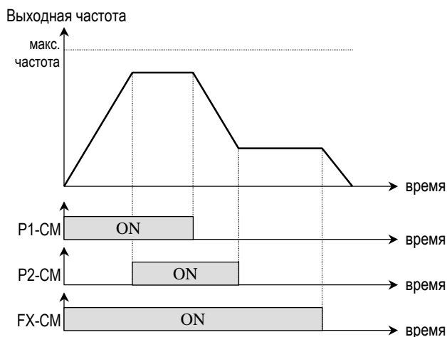
[Работа привода в режиме управления двумя кнопками Up/Down]
