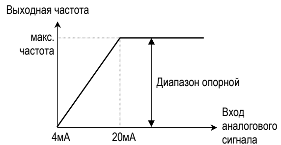
[Режим V-I: I (ток)]
