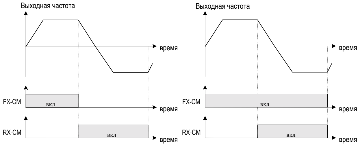
[FUN 02 - Управление Terminal-1 ]
