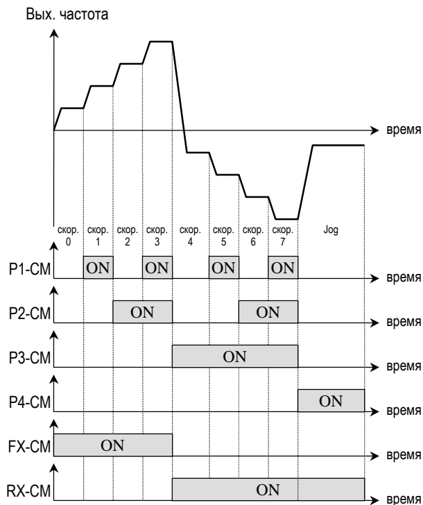
[Многоскоростной привод]
