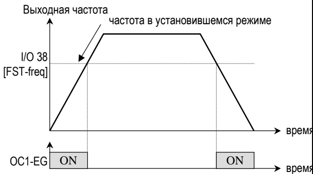
[Выход OC1 определен как 'FST-LO']
