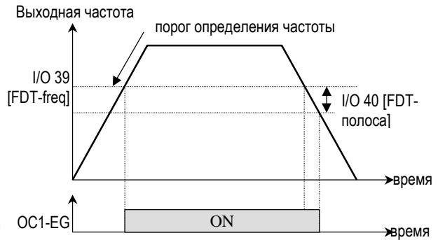
[Выход OC1 определен как 'FDT-HI']
