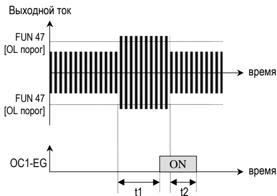
[Выход OC1 определен как 'OL']
