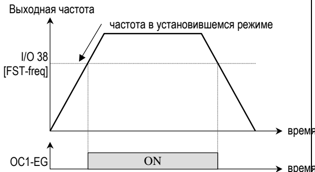
[Выход OC1 определен как 'FST-HI']
