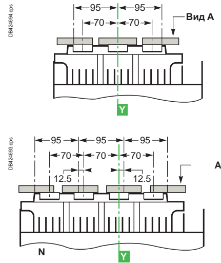
Левая или правая контактная пластина для 3-полюсного аппарата
