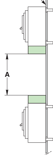
Заднее присоединение или цоколь аппаратов с короткими клеммными крышками
