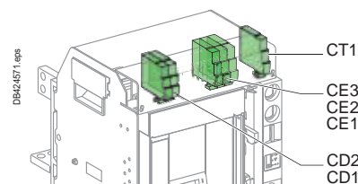
Выкатной аппарат
