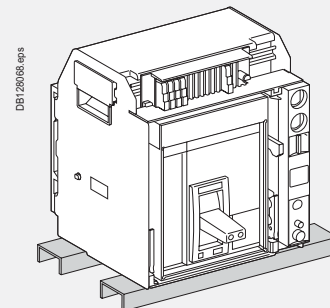
Нижнее крепление на металлоконструкции
