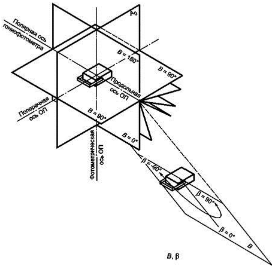
Рисунок Б.1 - Системы фотометрирования, лист 1
