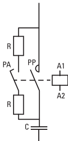
Рис. 1 Электрическая принципиальная схема КМЗК
