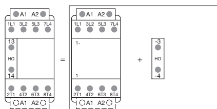
Комбинация 10 = AF09–AF80...-40-00 + CA4-10
