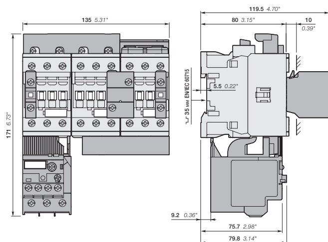
AF26, AF30, AF38 + BEY38-4, VEM4, CA4-10 + тепловое реле перегрузки TF42
