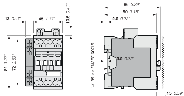
AF26..K, AF30..K, AF38..K + двухполюсный блок дополнительных контактов CAL4-11K
