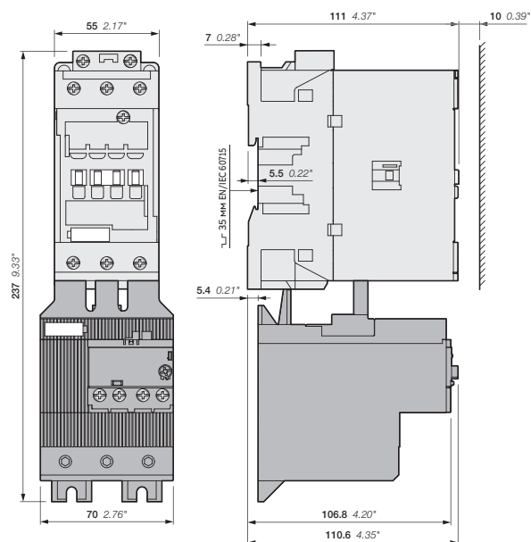
AF40, AF52, AF65 + электронное реле перегрузки EF65
