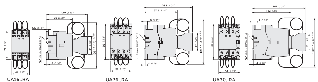
Основные габаритные размеры в мм и дюймах
