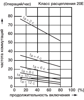
Класс расцепления 20E
