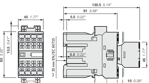
NFZ44EK, NFZ53EK, NFZ62EK, NFZ71EK, NFZ80EK
