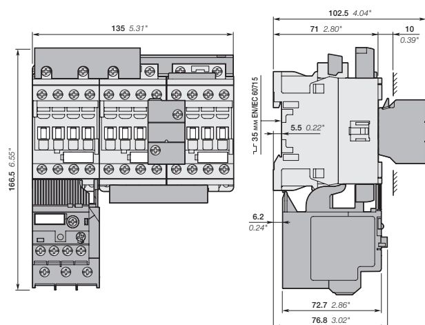
AF09, AF12, AF16 + BEY16-4, VEM4 + тепловое реле перегрузки TF42
