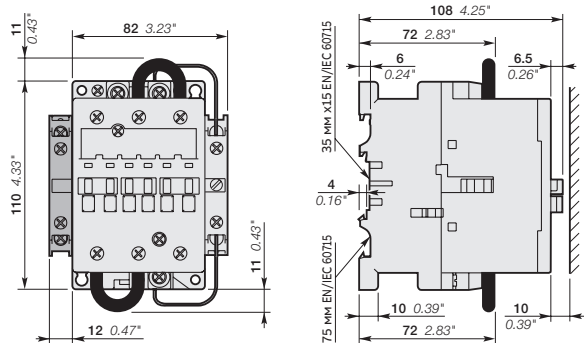
GAE75-10-11 Основные габаритные размеры в мм и дюймах
