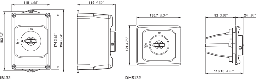
Основные габаритные размеры в мм и дюймах
