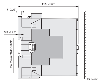
AF80, AF96-30-00 + двухполюсный блок дополнительных контактов CAL4-11 AF80, AF96-30-11
