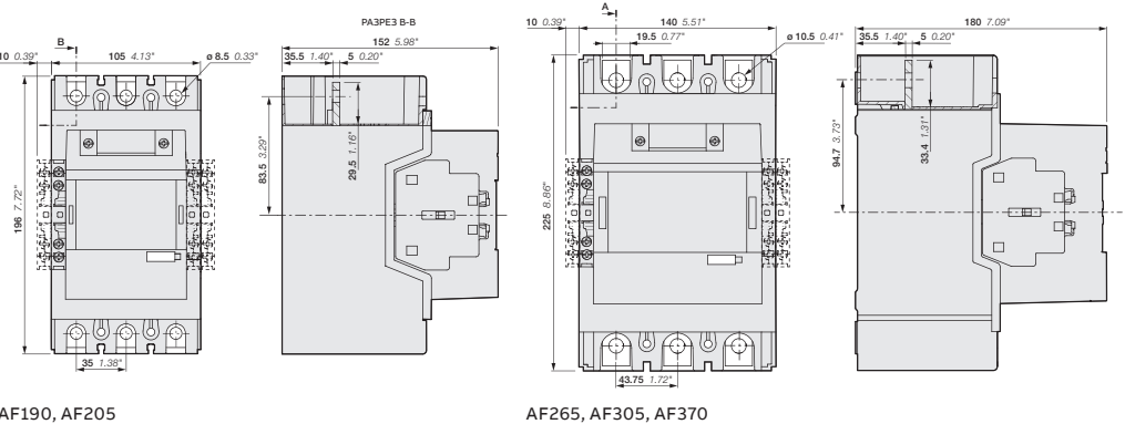
Основные габаритные размеры в мм и дюймах
