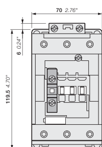
AF80, AF96 + однополюсный блок дополнительных контактов CA4, CC4
