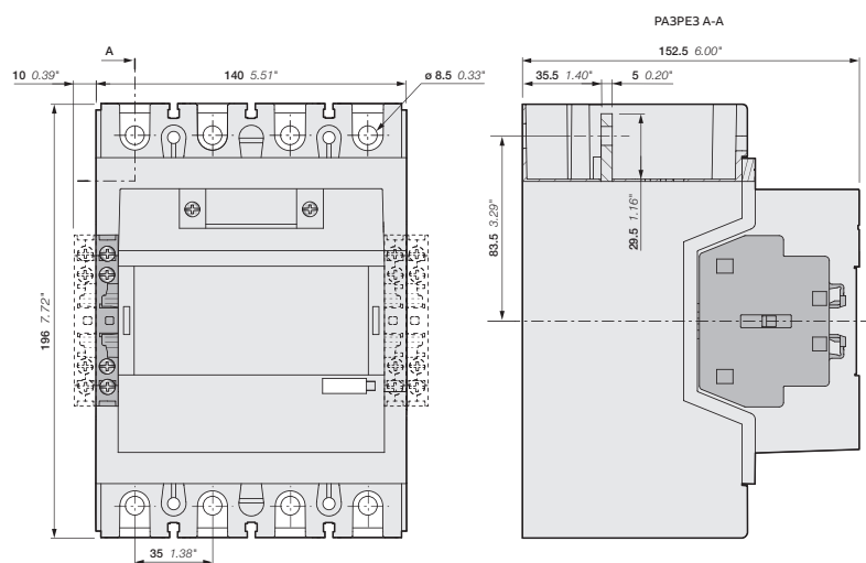
AF190, AF205-40-00 + двухполюсный блок дополнительных контактов CAL19 AF190, AF205-40-11
