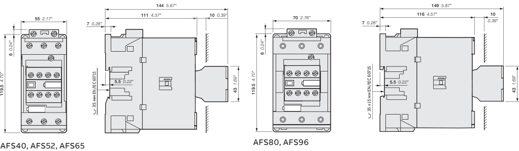
Основные габаритные размеры в мм и дюймах
