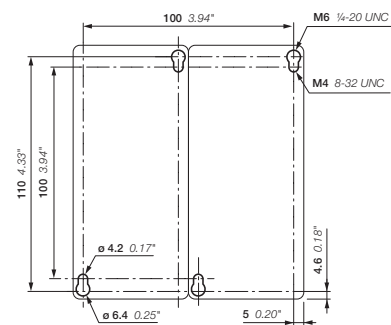
AF40, AF52, AF65 + механическая блокировка VM96-4
