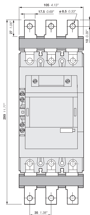
AF190, AF205-30-11 + удлинитель выводов LX205
