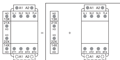
Комбинация 11 = CAL4-11 + AF09–AF80...-40-00
