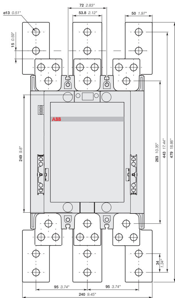
AF1250-30-11 + расширитель выводов LW1250
