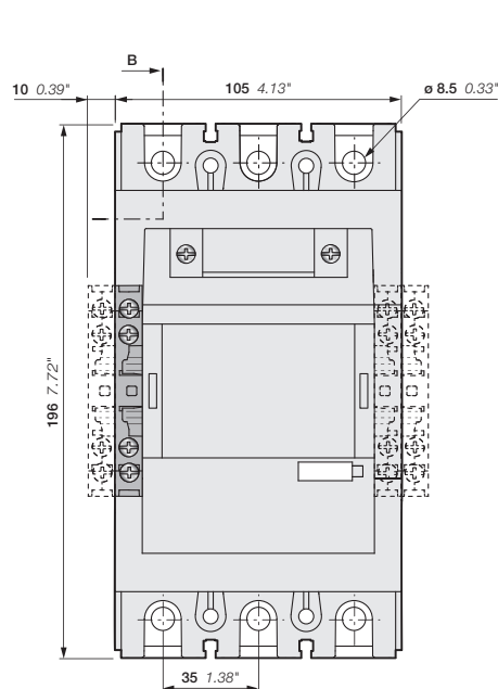
AF190, AF205-30-00 + двухполюсный блок дополнительных контактов CAL19 AF190, AF205-30-11
