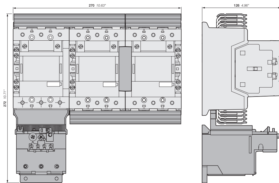
AF116, AF140, AF146 + BEY140-4, VM19 + тепловое реле перегрузки TF140
