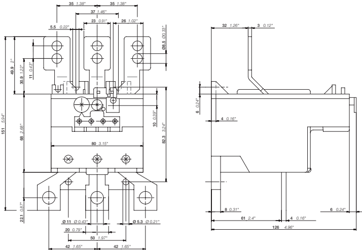
Основные габаритные размеры в мм и дюймах
