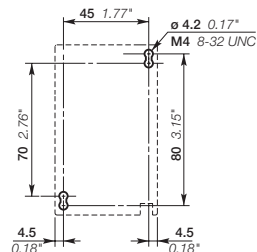
Схема монтажных отверстий для UA26, UA30
