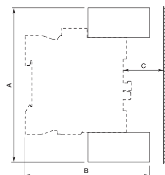
Основные габаритные размеры
