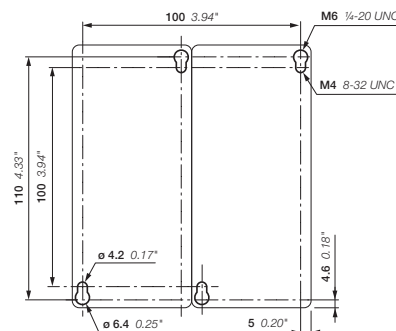
AF40, AF52, AF65 + BER65-4, VM96-4 + электронное реле перегрузки EF65
