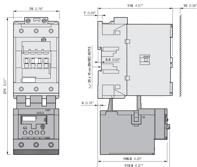
AF80, AF96 + тепловое реле перегрузки TF96
