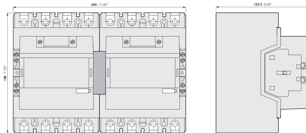
AF190, AF205-40-11 + механическая блокировка VM19
