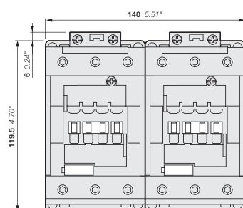
AF80, AF96 + механическая блокировка VM96-4
