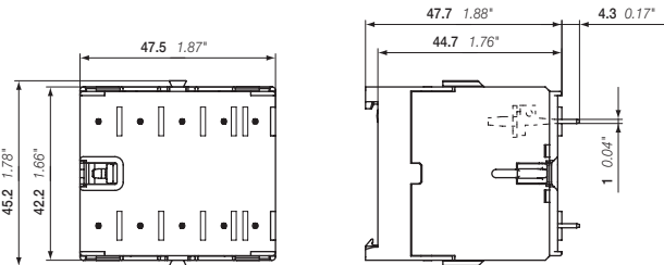
K6 Основные габаритные размеры в мм и дюймах
