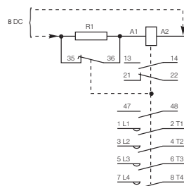
ЕК550, ЕК1000 с катушкой управления DC
