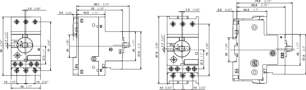
MS116 ≤ 16 А с установленным блоком доп. контактов НКФ1 MS116 ≥ 20 А с установленным блоком доп. контактов НКФ1
