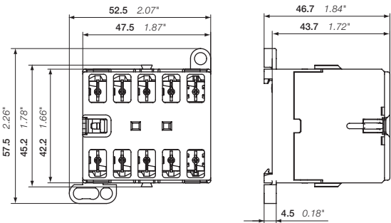
K6 Основные габаритные размеры в мм и дюймах
