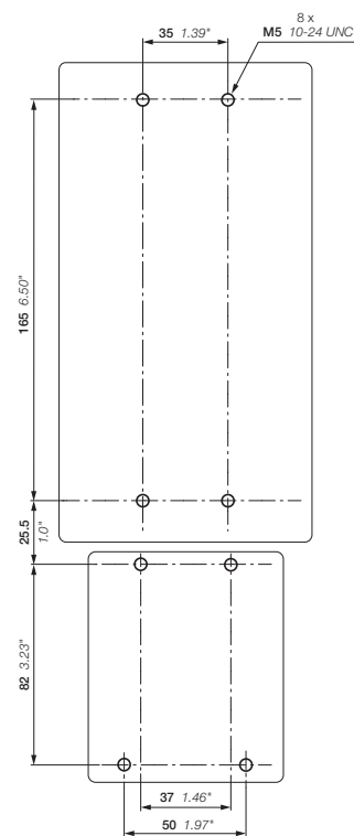
AF190, AF205 + тепловое реле перегрузки TA200DU
