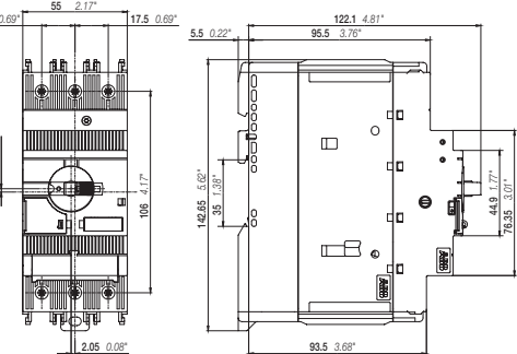
MS165 Основные габаритные размеры в мм и дюймах
