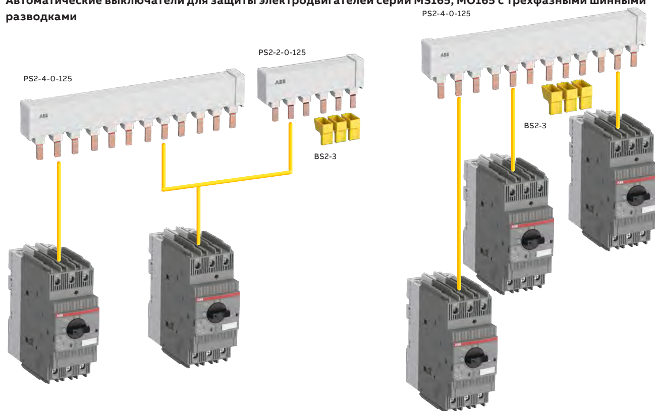
Трехфазная шинная разводка до 125 А
