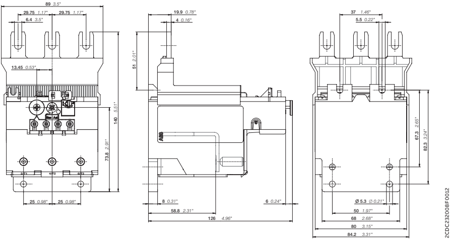
Основные габаритные размеры в мм и дюймах
