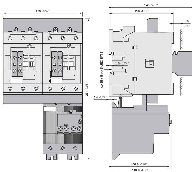
AF80, AF96 + BER96-4, VM96-4 + электронное реле перегрузки EF96
