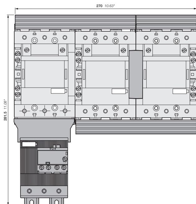
AF116, AF140, AF146 + BEY140-4, VM19 + электронное реле перегрузки EF146
