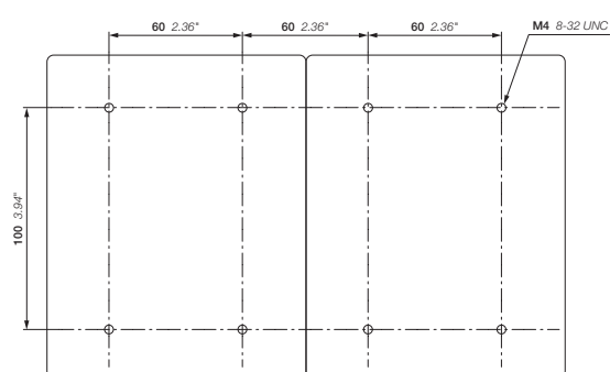
AF116, AF140 + механическая блокировка VM19
