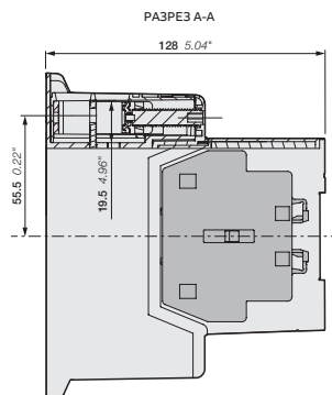
AF116, AF140-40-00 + двухполюсный блок дополнительных контактов CAL19 AF116, AF140-40-11
