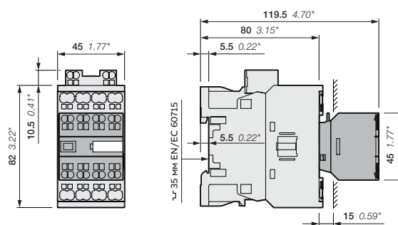
AF26..K, AF30..K, AF38..K + четырехполюсный блок дополнительных контактов CA4..K
