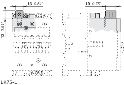
Основные габаритные размеры в мм и дюймах
