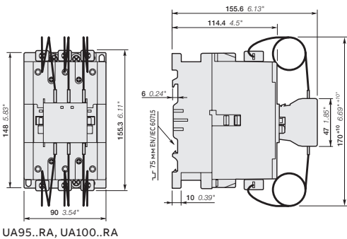
Основные габаритные размеры в мм и дюймах
