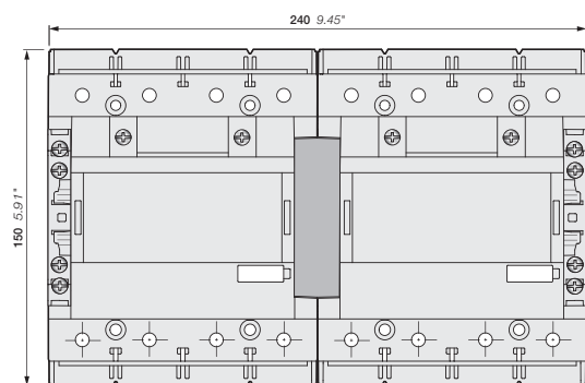
AF116, AF140-40-11 + механическая блокировка VM19
