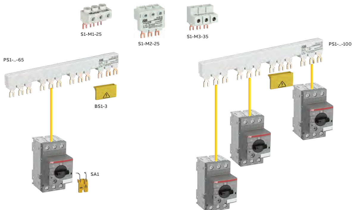
Трехфазная шинная разводка до 65 А
