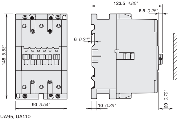
Основные габаритные размеры в мм и дюймах
