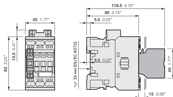
AF26..K, AF30..K, AF38..K + однополюсный блок дополнительных контактов CA4..K
