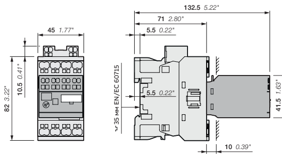
AF09..K, AF12..K, AF16..K + электронная приставка времени TEF4S
