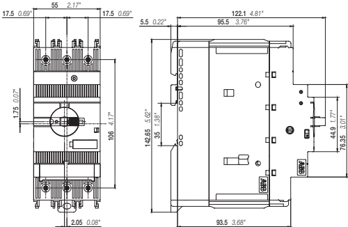
MO165 Основные габаритные размеры в мм и дюймах
