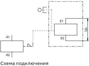
Схема подключения
