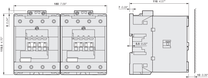
AF80 + однополюсный блок дополнительных контактов CA4, CC4
