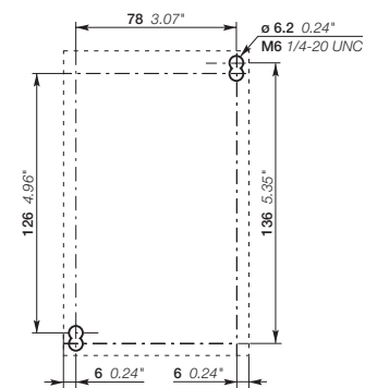
Схема монтажных отверстий
