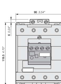
AF80 + электронная приставка времени TEF4
