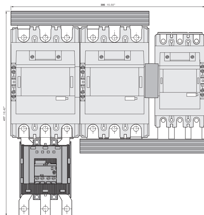
Линия, треугольник: AF265, AF305, AF370 + звезда: AF190, AF205 + BEY265-4, VM205/265 + электронное реле перегрузки EF370
