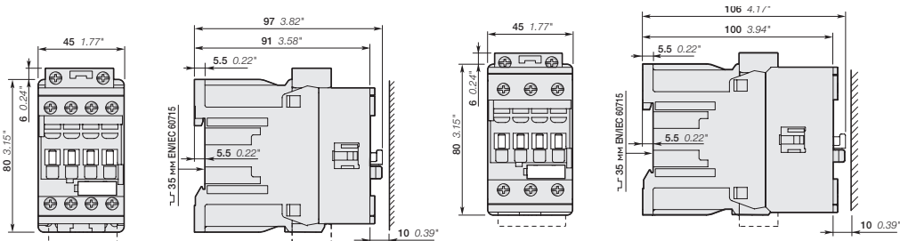
AF26Z, AF30Z, AF38Z
