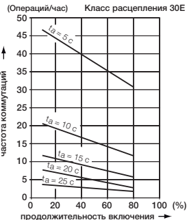
Класс расцепления 30E
