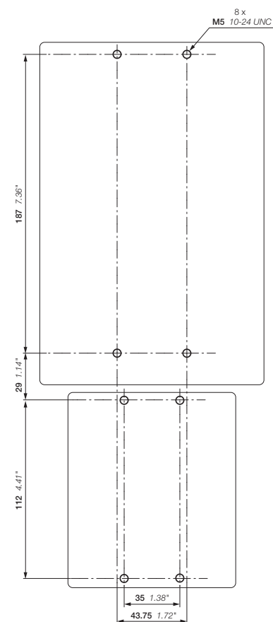
AF265, AF305, AF370 + электронное реле перегрузки EF370
