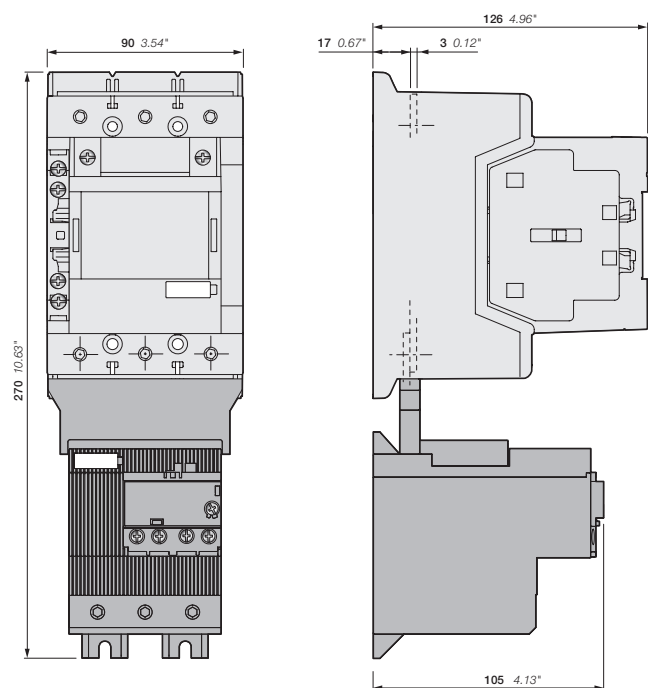
AF116, AF140, AF146-30-11 + электронное реле перегрузки EF146
