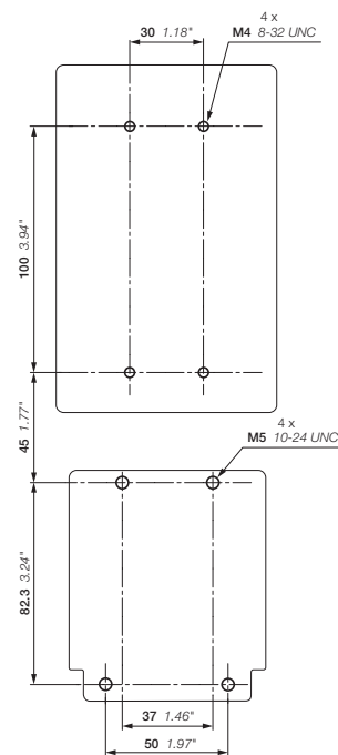
AF116, AF140-30-11(B) + тепловое реле перегрузки TF140
