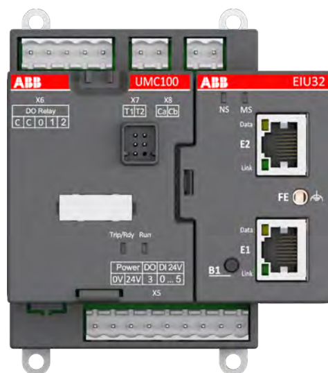
Универсальный контроллер электродвигателя UMC100.3 с интерфейсом EtherNet/IP™ EIU32.0
