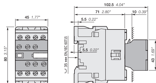
AF09, AF12, AF16 + двухполюсный дополнительный контакт CAT4 с фронтальной клеммой катушки
