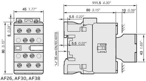
Основные габаритные размеры в мм и дюймах
