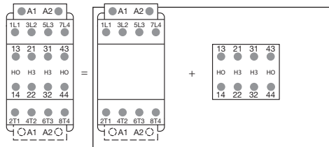
Комбинация 22 = AF09–AF80...-40-00 + CA4-22E
