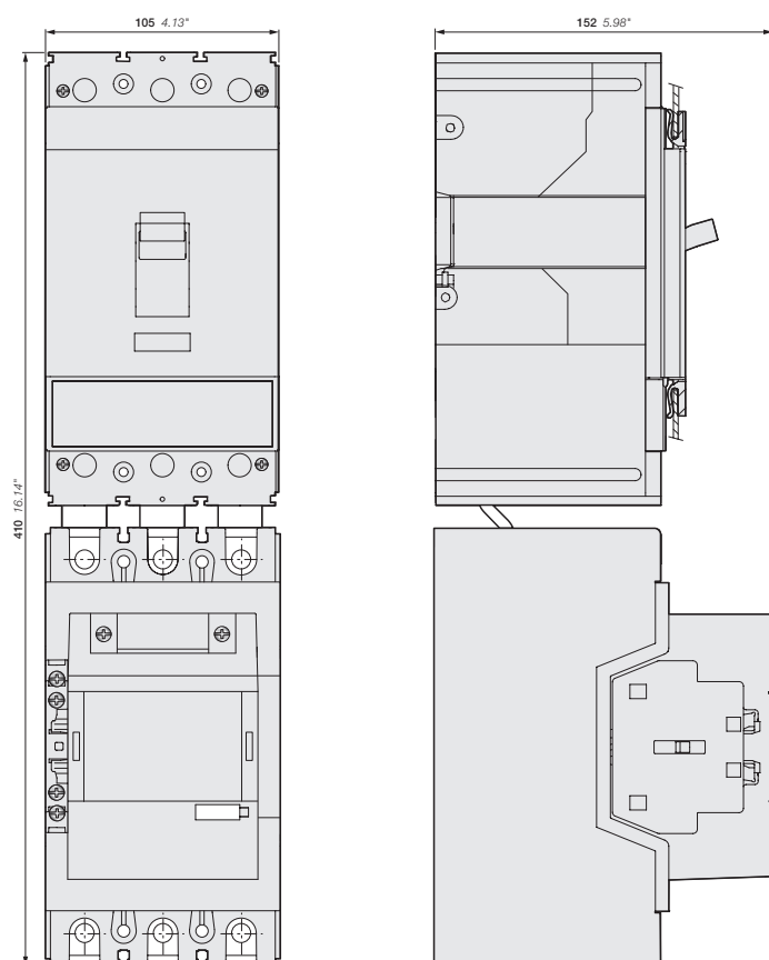
T4S + BEA205/T4 + AF190, AF205
