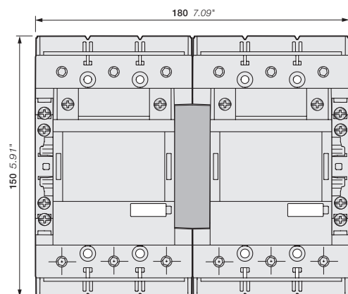
AF116, AF140, AF146-30-11 + механическая блокировка VM19
