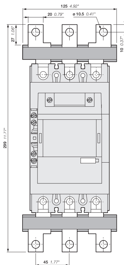
AF190, AF205-30-11 + расширитель выводов LW205
