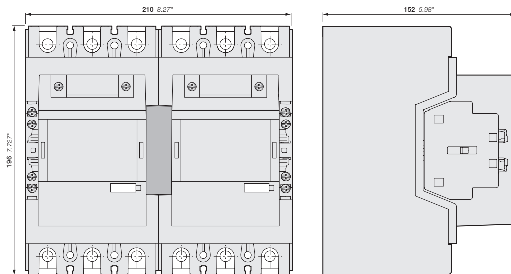
AF190, AF205-30-11 + механическая блокировка VM19
