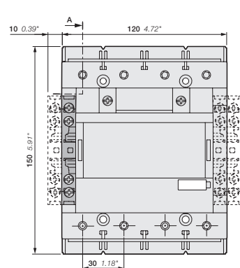
AF116, AF140-40-00 + двухполюсный блок дополнительных контактов CAL19 AF116, AF140-40-11
