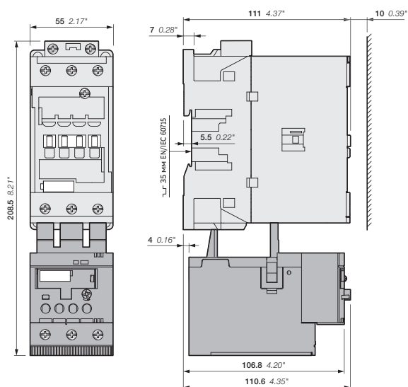
AF40, AF52, AF65 + тепловое реле перегрузки TF65
