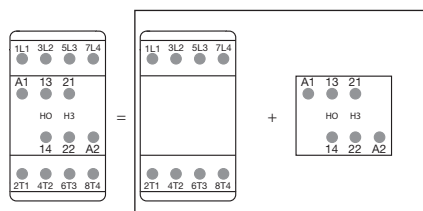
Комбинация 11 = AF09–AF80...-40-00 + CAT4-11E
