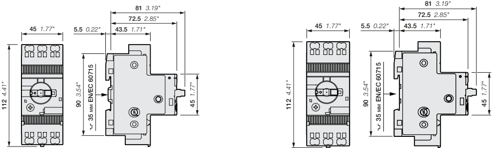
MS132-K > 10 А MS132-K ≤ 10 А
