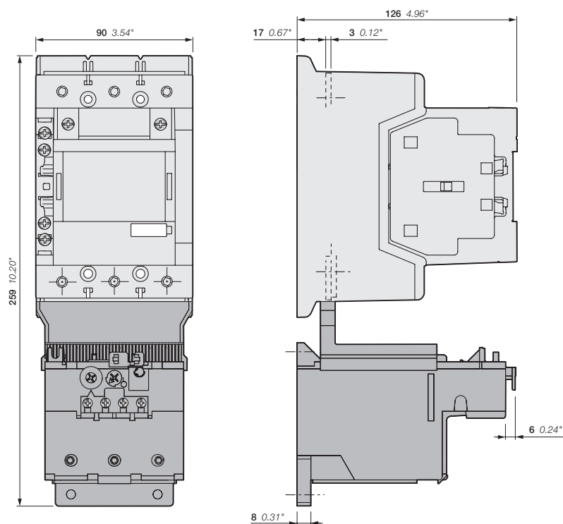
AF116, AF140-30-11 + тепловое реле перегрузки TF140
