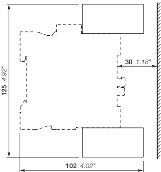
Основные габаритные размеры в мм и дюймах
