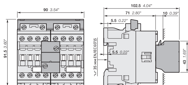
AF09..-40-00, AF16..-40-00 + электромеханическая блокировка VEM4
