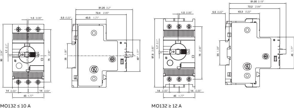
Основные габаритные размеры в мм и дюймах
