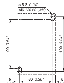
Схема монтажных отверстий
