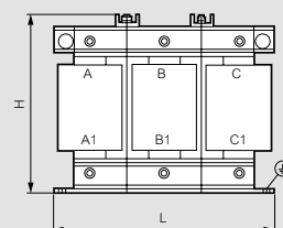
Для подключения алюминиевых шин
