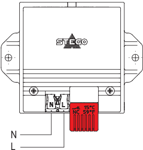
Пример подключения нагревателя с вентилятором CSF 028
