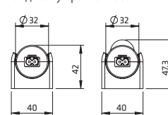
Вид сбоку Крепление зажимом
