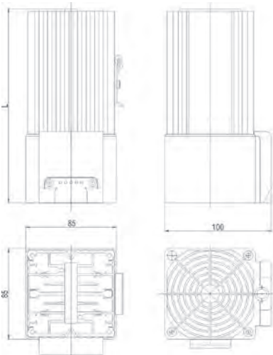
Нагреватель с вентилятором HGL 046
