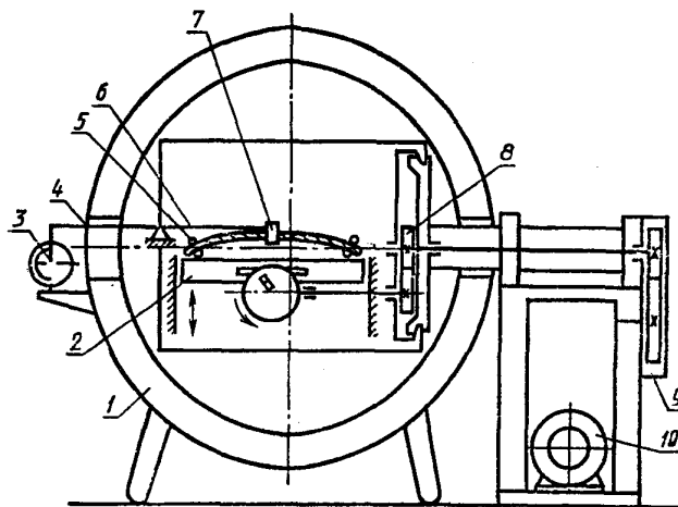
Схема стенда для определения усилия изгиба кабеля
