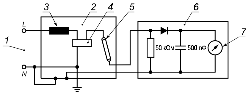
1 — сеть; 2 — светильник; 3 — ПРА; 4 — зажигающее устройство; 5 — лампа; 6 — измерительное устройство; 7 — высоко- омный вольтметр
