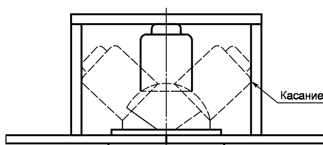
Вращение светильника на 350°
