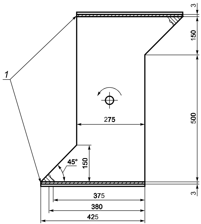
1 — стальная пластина
