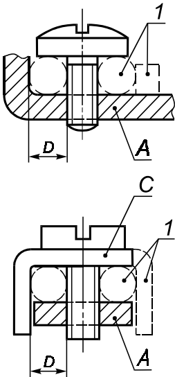
Винт, не требующий шайбы или прижимной пластины
