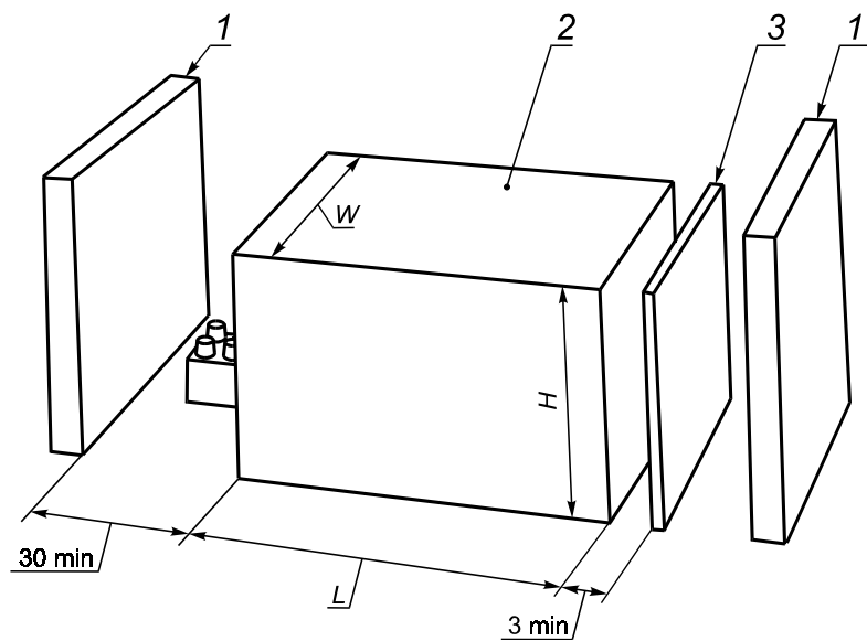
1 — воспламеняемый материал; 2 — ПРА; 3 — экран
