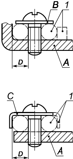
Винт, требующий шайбу или прижимную пластину
