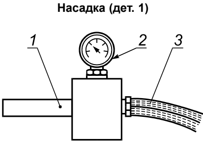
1 — насадка; 2 — манометр; 3 — шланг
