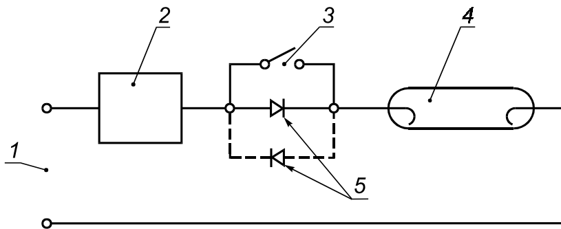
1 — сеть; 2 — испытываемый ПРА; 3 — выключатель; 4 — лампа; 5 — выпрямитель
